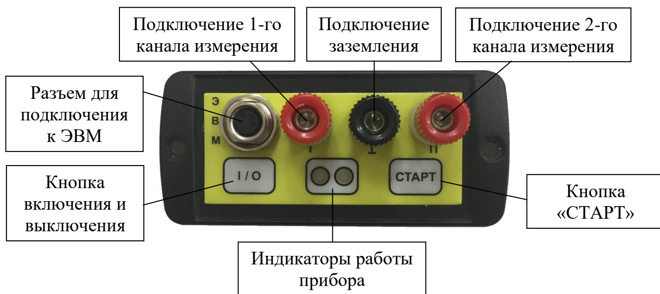
Рисунок 1 – Лицевая панель Регистратора
